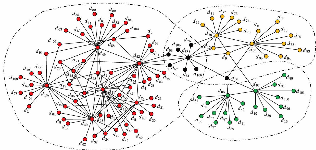
Fig. 8 The semantic community of QLSP network. 图 8 QLSP 网络语义社区划分结果
