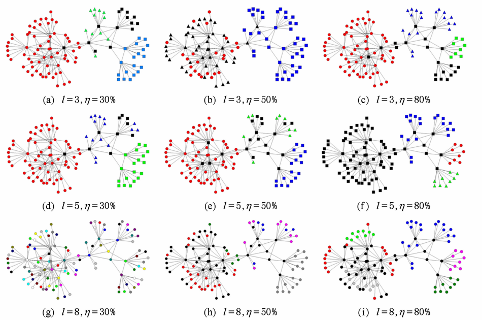
Fig. 9 Community structures with different l and \eta . 图 9 l 和 \eta 在不同取值下的网络划分结果
