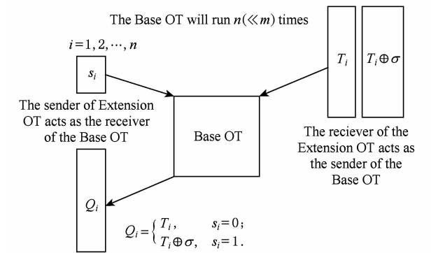
Fig. 8 The map of first stage. 图 8 第 1 阶段示意图
