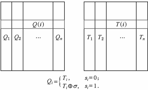
Fig. 9 Result of Base OT. 图 9 基础 OT 执行结果
