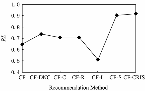
Fig. 4 Comparison of recall (RL) using Epinions dataset. 图4 采用 Epinions 数据集召回率(RL)对比
