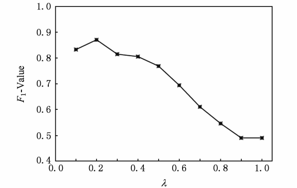
Fig. 3 F_1 -values under different \lambda on training corpus. 图 3 F_1 值与参数 \lambda 在训练集上的关系
