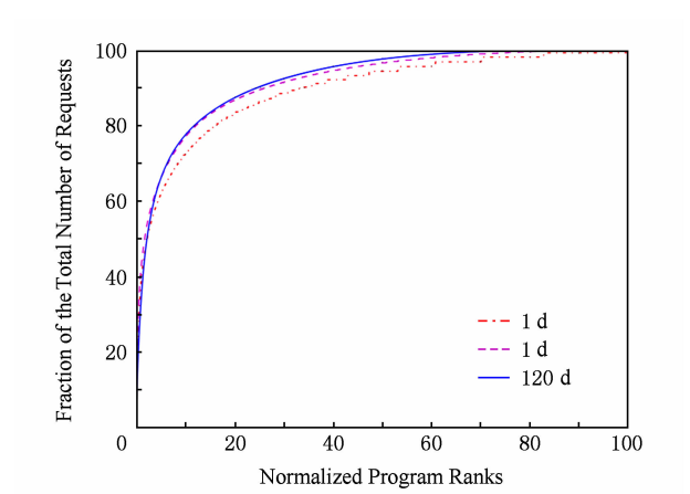
Fig. 3 Cumulative distribution of requests to programs. 图 3 收视次数随节目排名的累积分布
