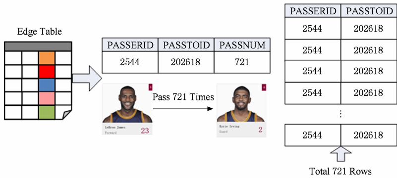
Fig. 4 Input data transformation for PR computing. 图 4 PR 计算输入数据变换示例
