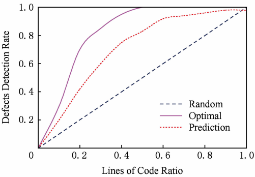
Fig. 2 CE cruve 图 2 CE 曲线
