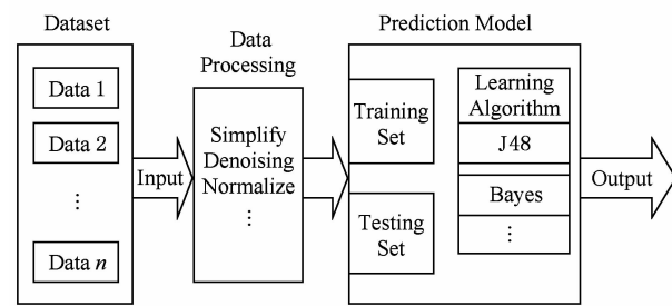
Fig. 1 Software defects prediction model 图 1 软件缺陷预测模型
