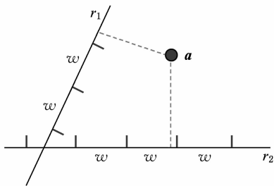
Fig. 1 p -stable distribution definition 图 1 p 稳定分布定义图
