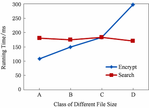
Fig. 7 Influence of file size 图 7 文件大小的影响
