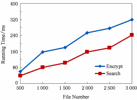
Fig. 8 Influence of file number 图 8 文件数量的影响
