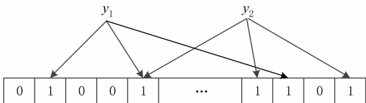
Fig. 2 The sample figure of Bloom filter 图 2 布隆过滤器示例图
