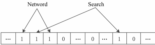
Fig. 5 Example of generating the trapdoor 图 5 生成陷门示例
