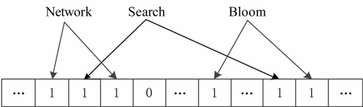
Fig. 4 Sample of generation security index 图 4 生成安全索引示例
