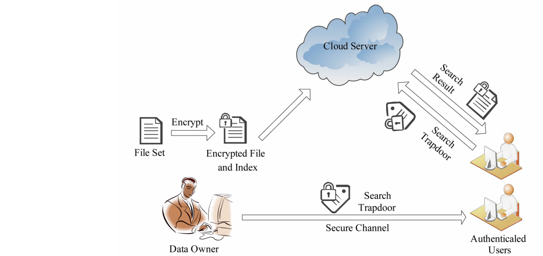
Fig. 3 Basic architecture 图 3 方案基本架构
