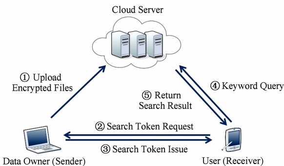
Fig. 1 Architecture of searchable encryption 图 1 可搜索加密基本框架
