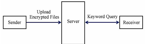
Fig. 2 One-to-one mode searchable encryption 图 2 一对一模式的可搜索加密
