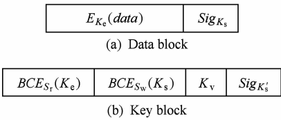
Fig. 2 Data format stored in the cloud 图 2 存储在云端的数据格式
