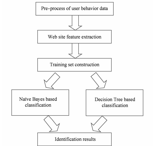
Fig. 5 Flowchart of identifying porn sites. 图 5 色情网站识别流程图
